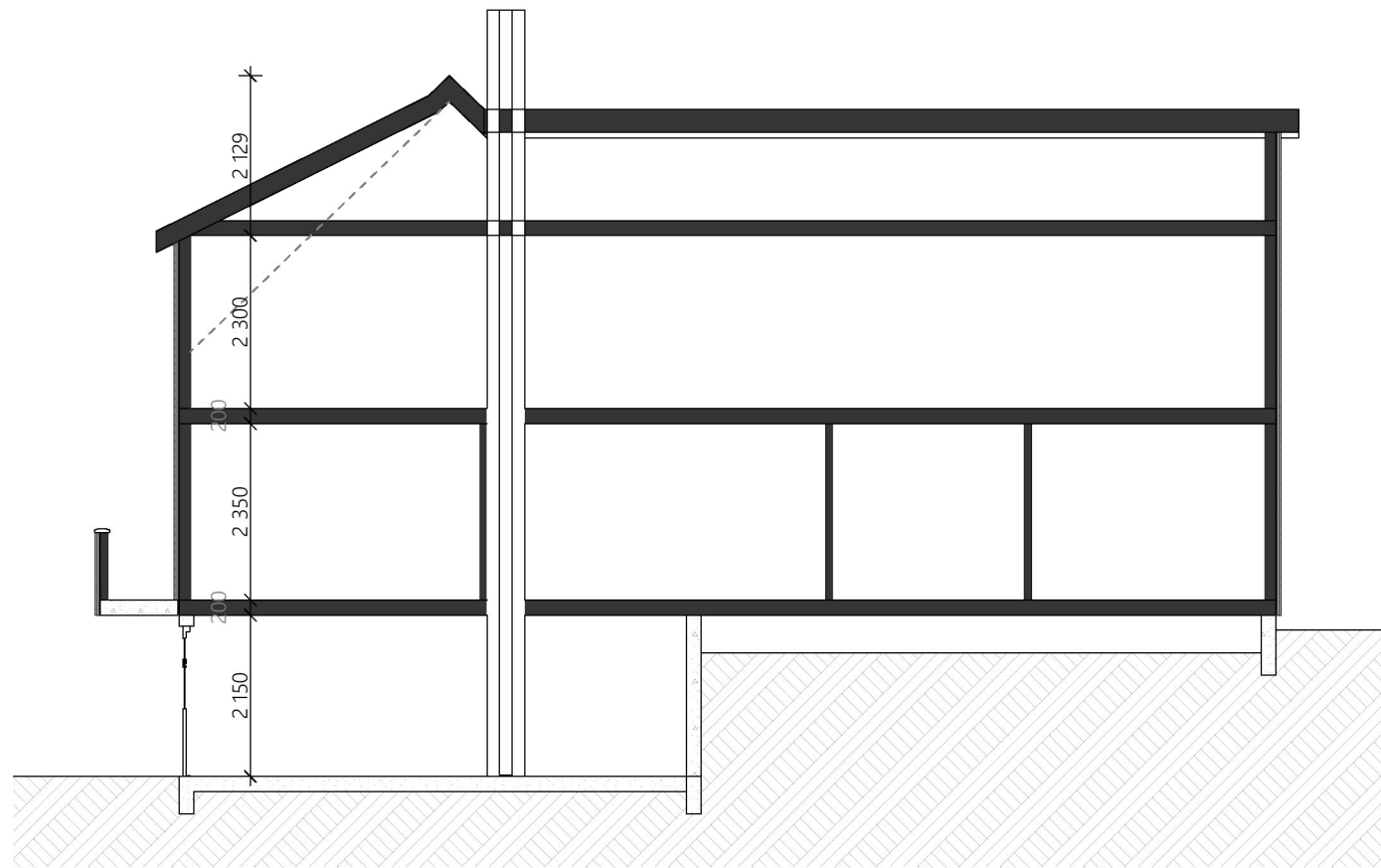
SNITT B-B
