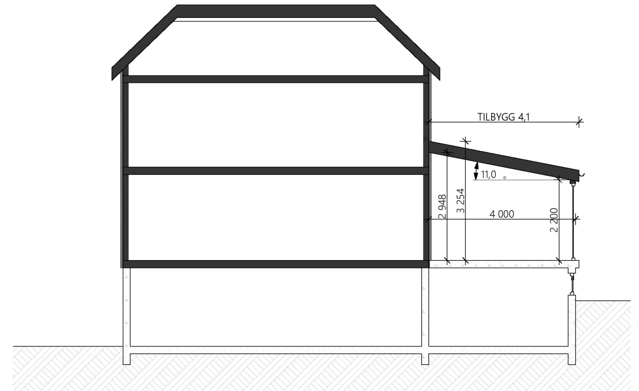
SNITT A-A
