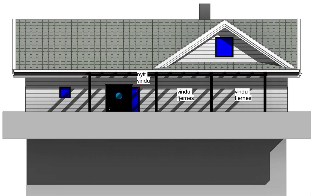
øst 1 : 100
