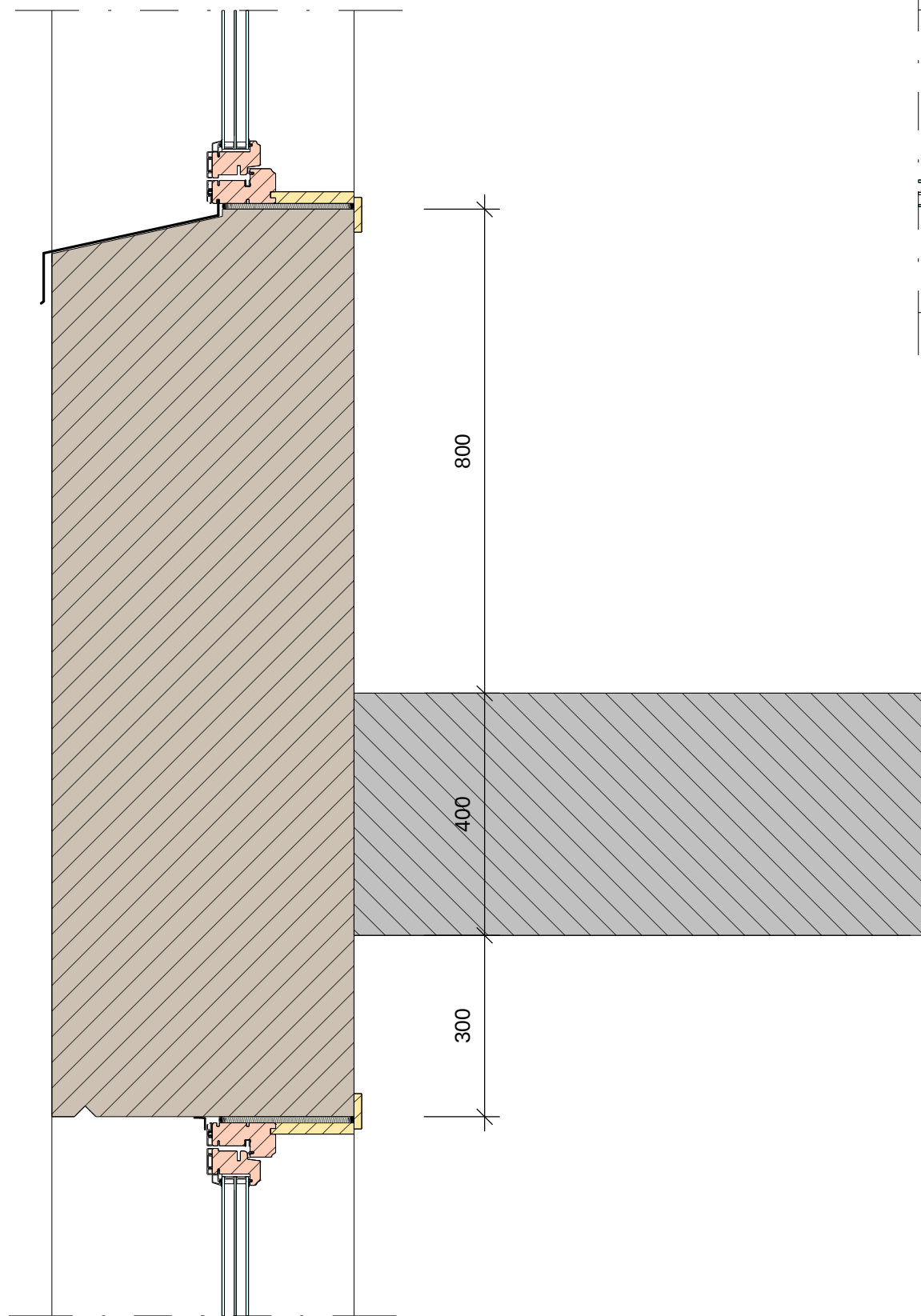
VERT. SNITT
