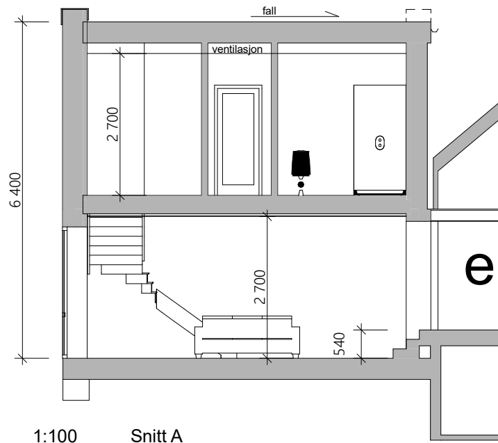
1:100 Snitt A
