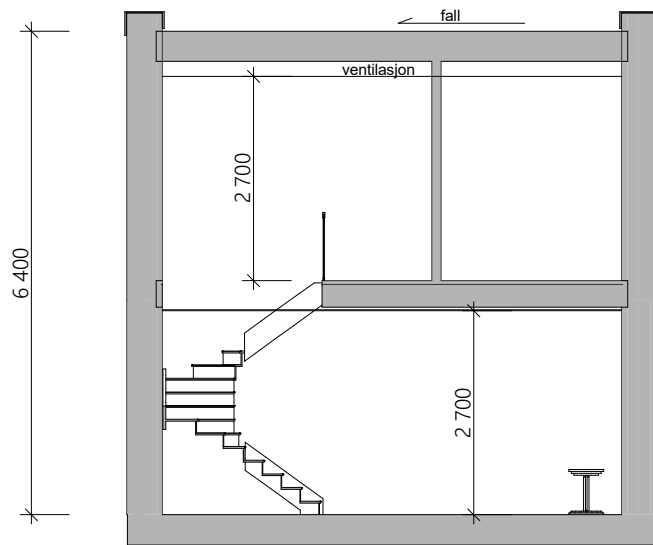
1:100 Snitt B
