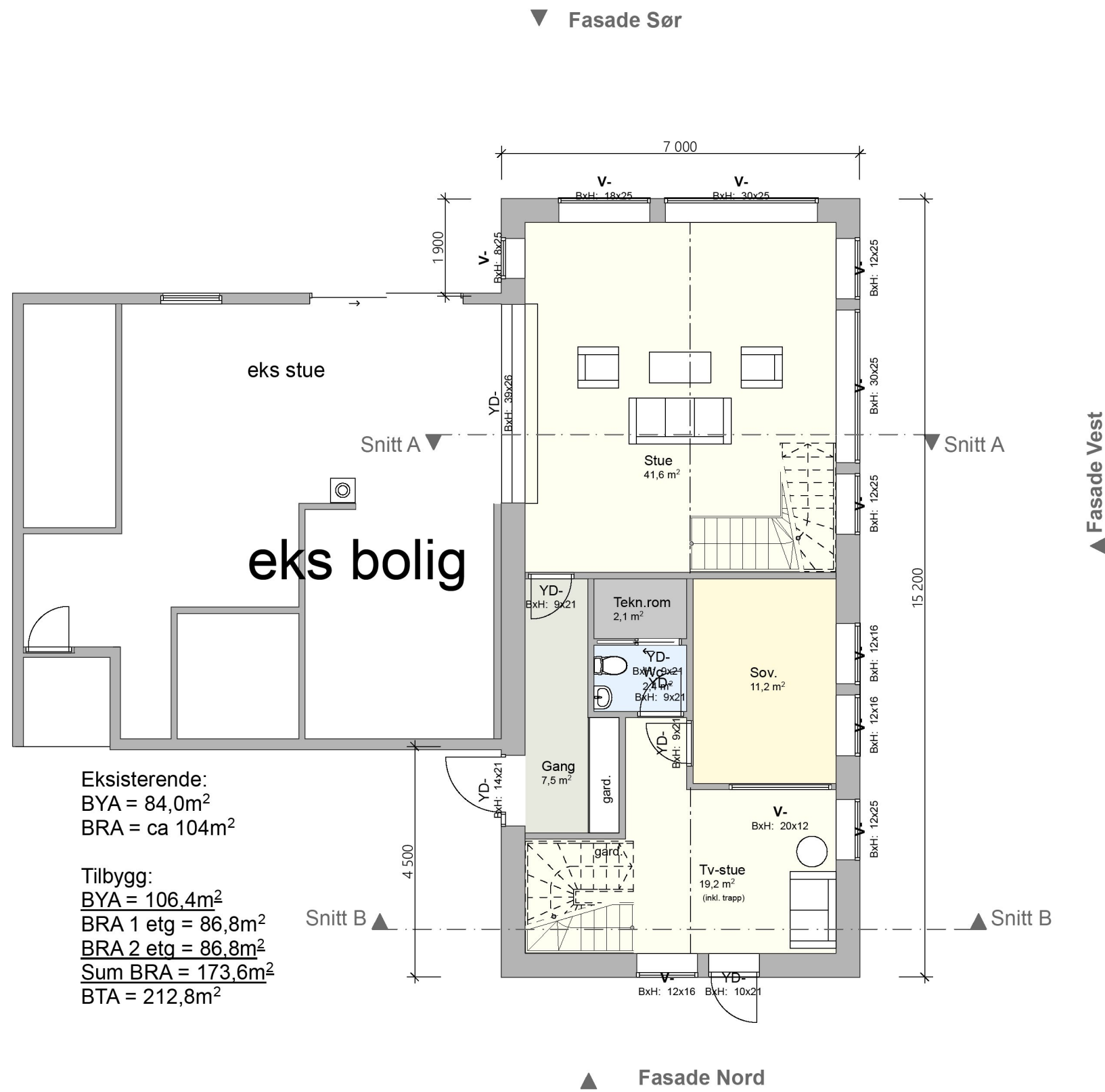
Plan 1 etg.
