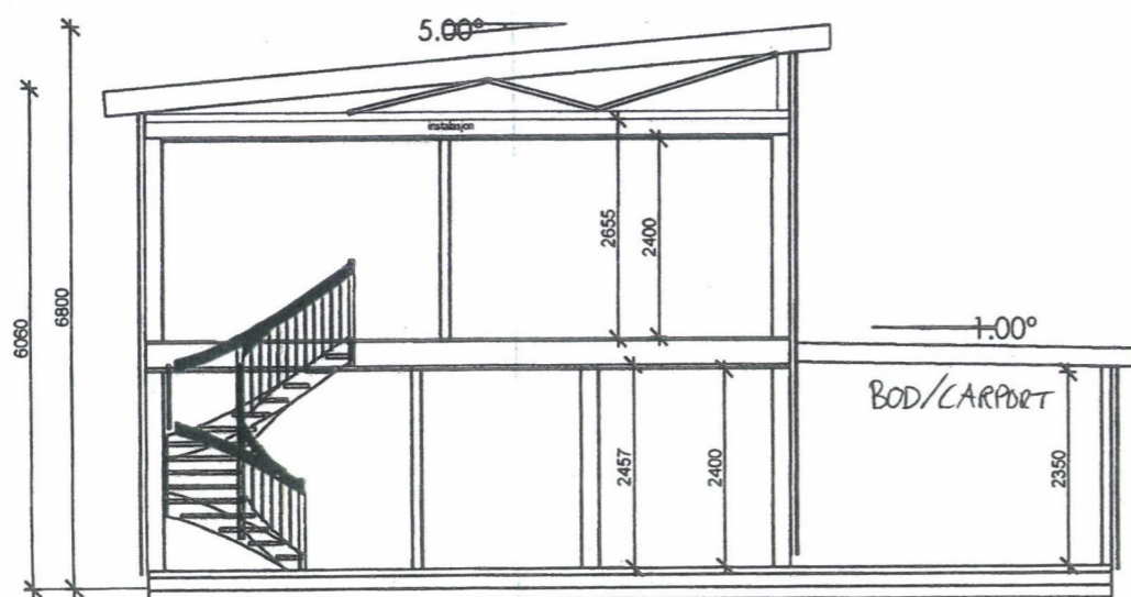
SNITT A-A
