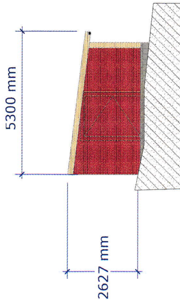
1 Fasade Vest Scale: 1:100
