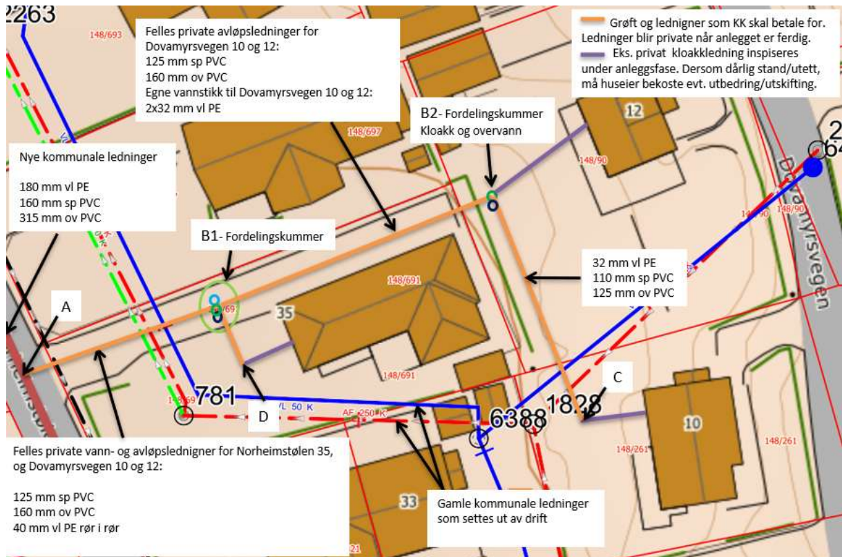
Prosjektert løsning for private stikkledninger Dovamyrsvegen 10, 12 og Norheimstølen 35.
