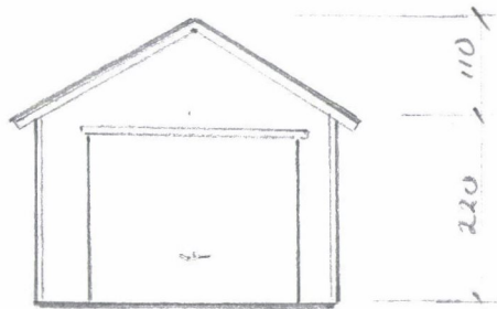
FASADE ØST
