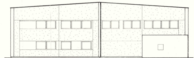
FASADE VEST
