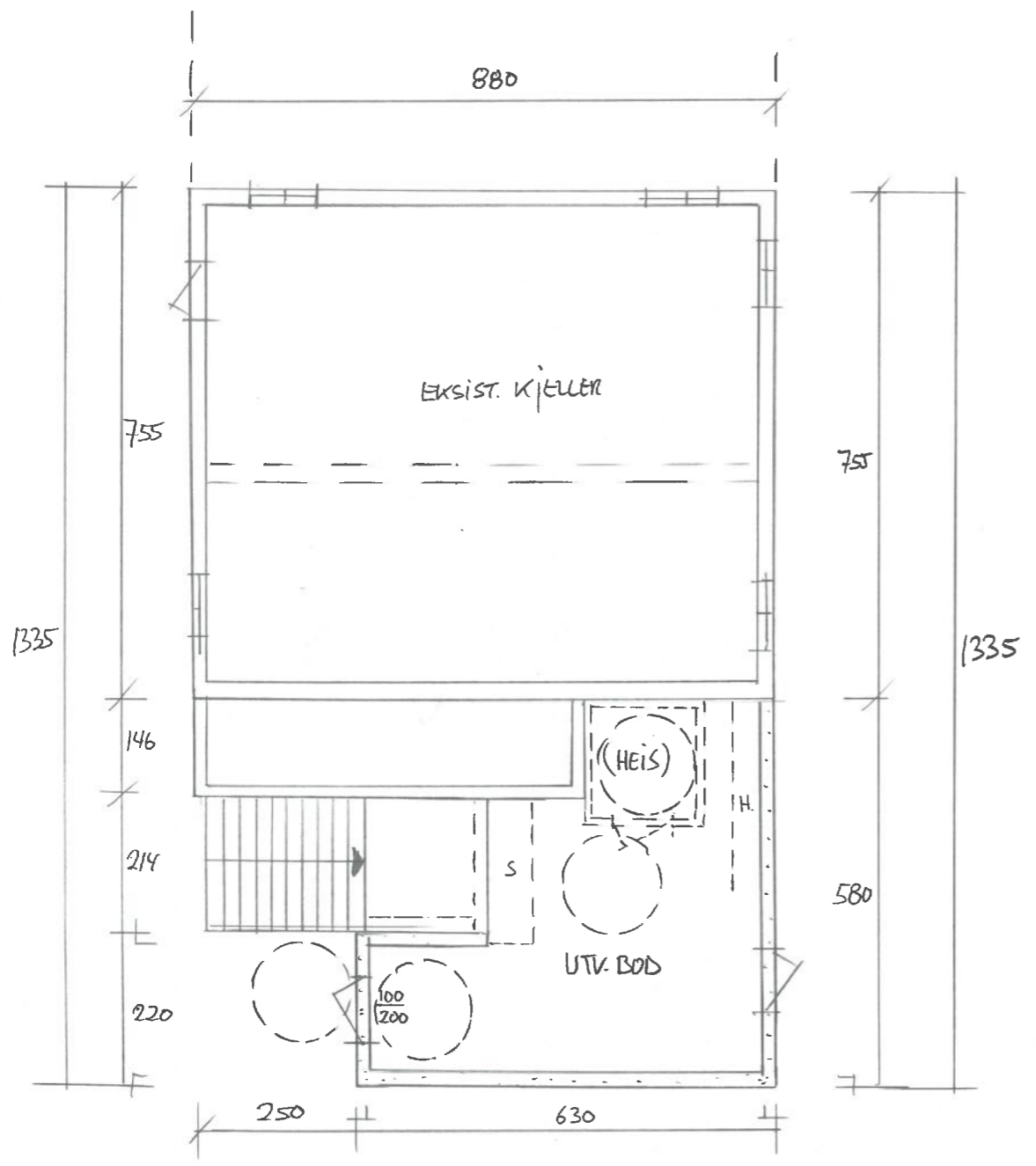
KJELLER PLAN
