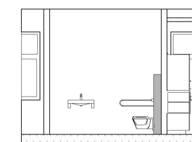
Snitt. Planlagt HCWC
