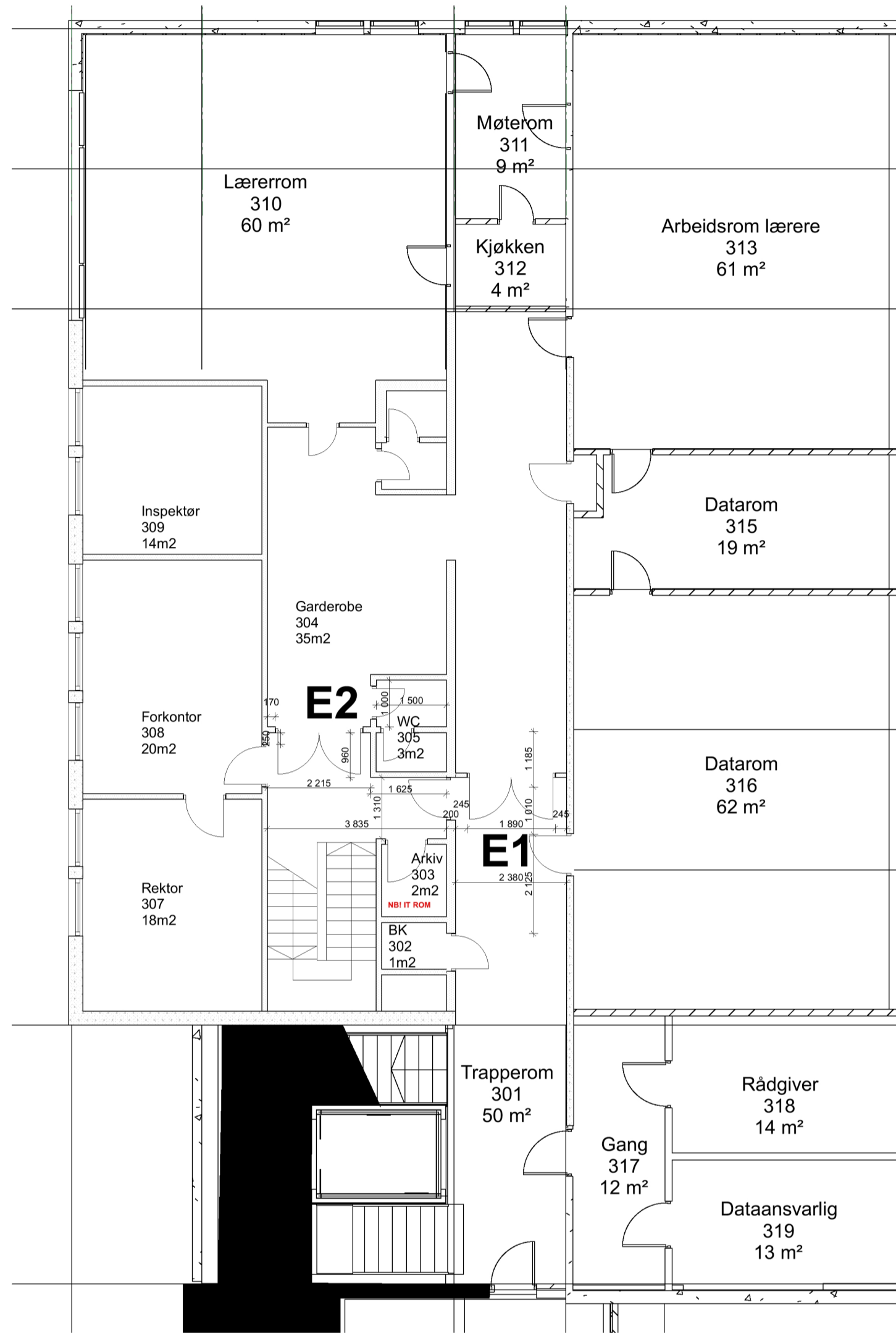
Eksisterende situasjon 3.etasje
