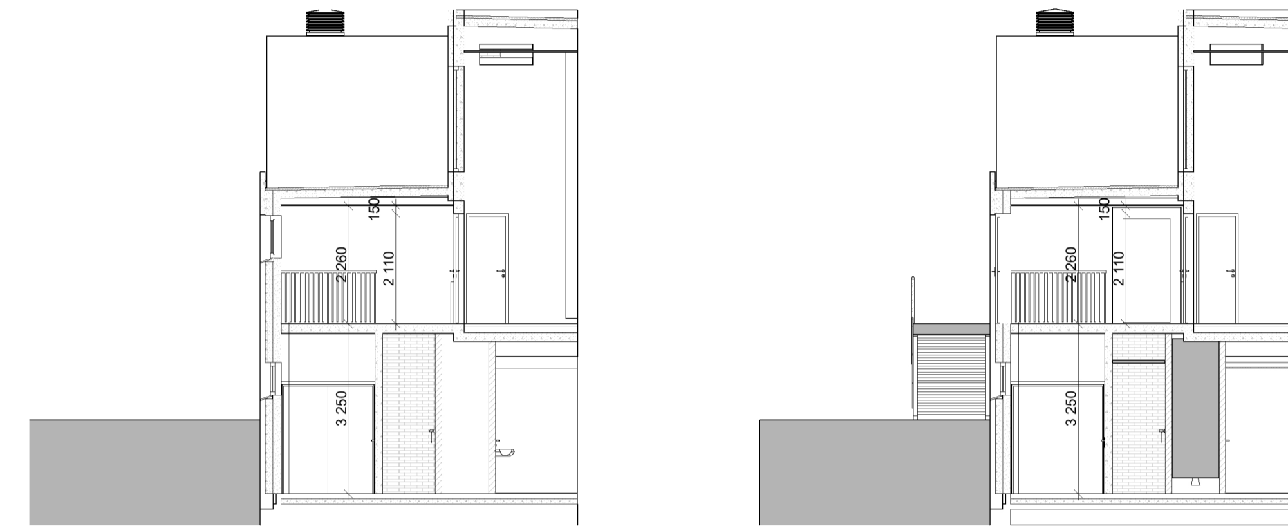
Snitt eksisterende situasjon
