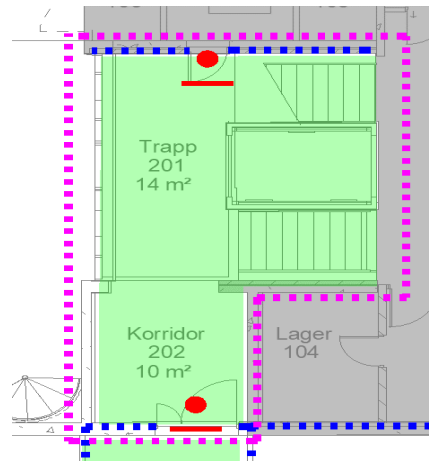
Figur 6: Omriss i lilla viser tiltaksgrense TEK 17 andre etasje
