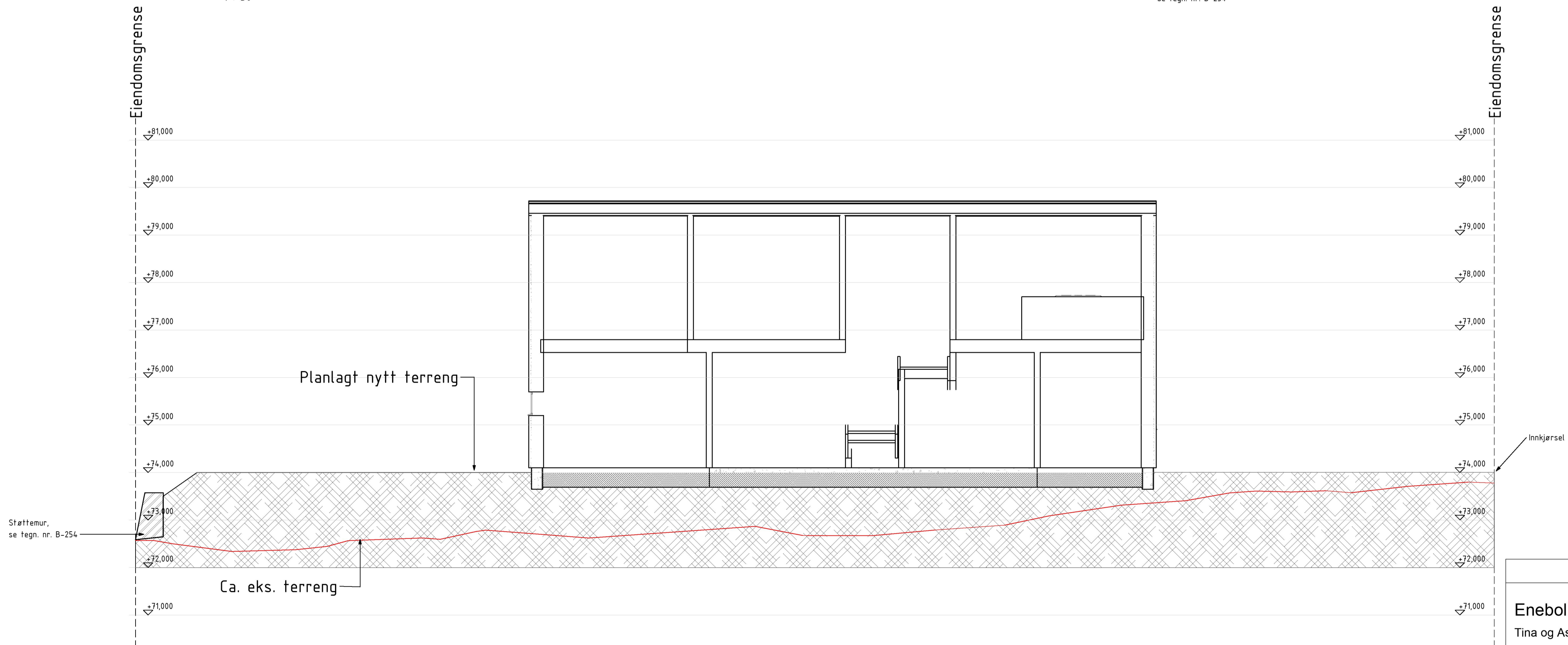
Terrenqsnitt 2 1 : 50
