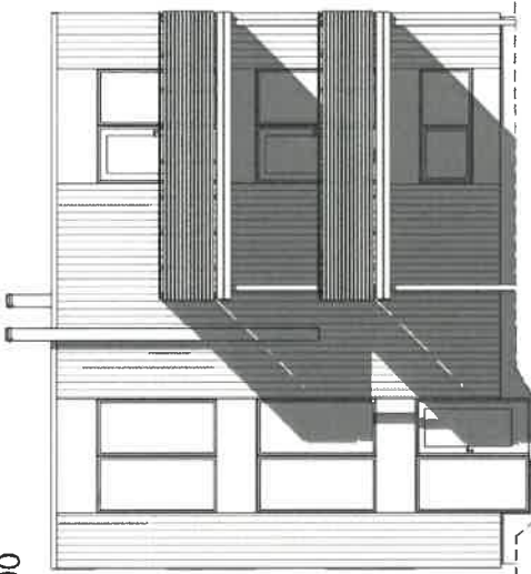
Øst 1 : 100
