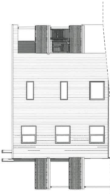
Øst 1 : 100
