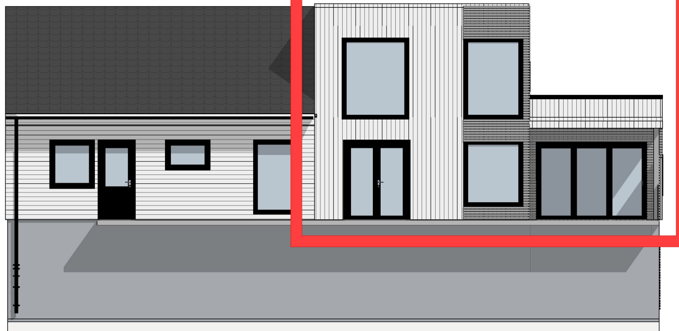
1:100 Fasade Sør
