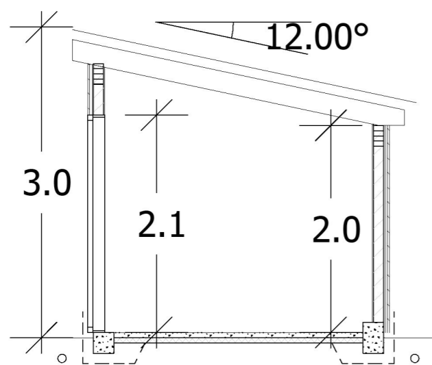
Snitt A-A
