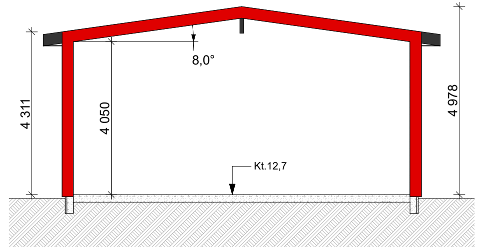
SNITT B-B
