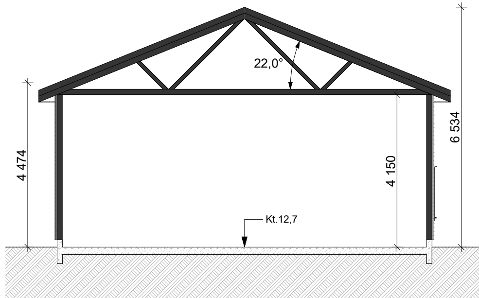
SNITT A-A
