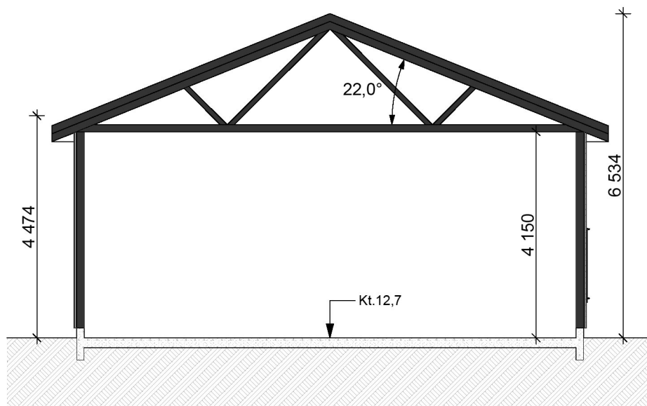
SNITT A
