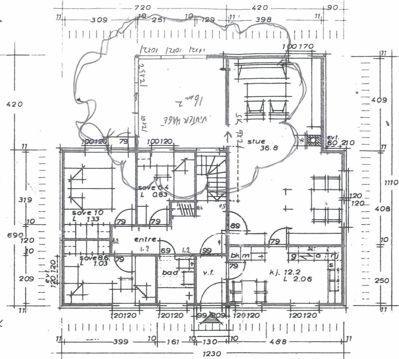
PLAN 1. ETG.
