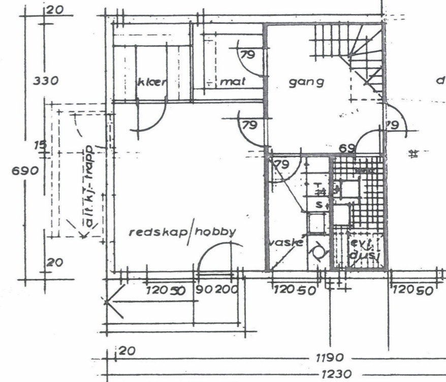
PLAN KJELLER
