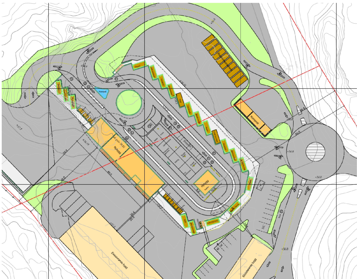
Figur: Situasjonsplan
