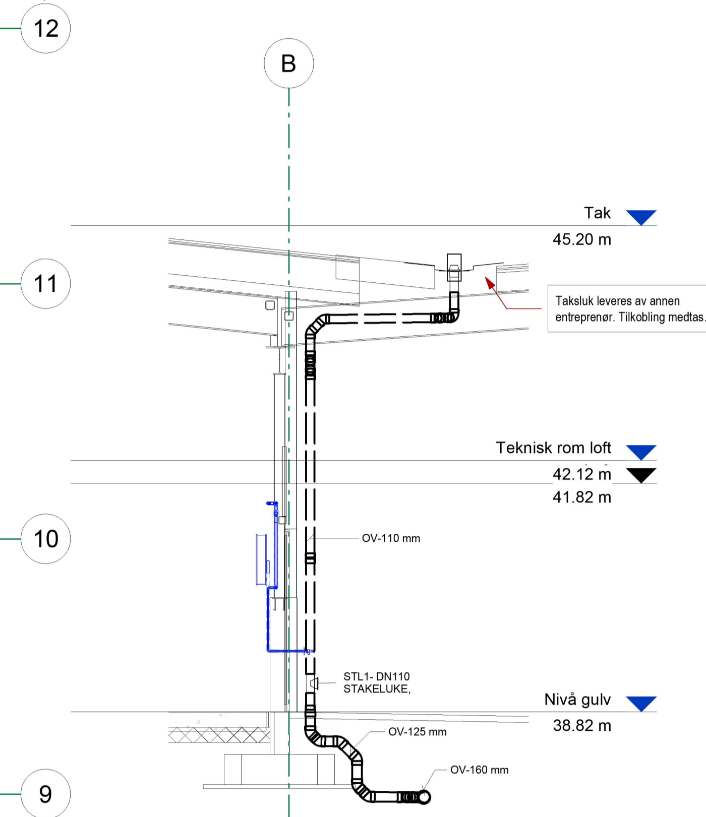
3 Prinsipp taksluk 1 : 50
