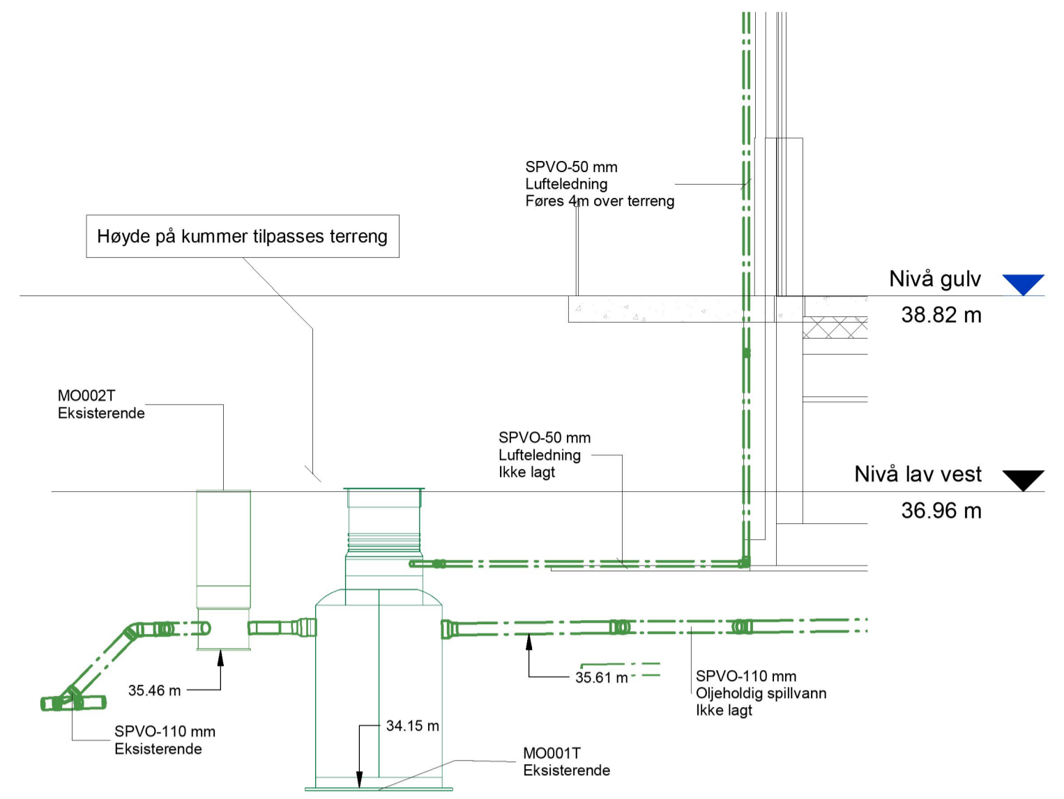
2 Snitt oljeutskiller 1 : 50
