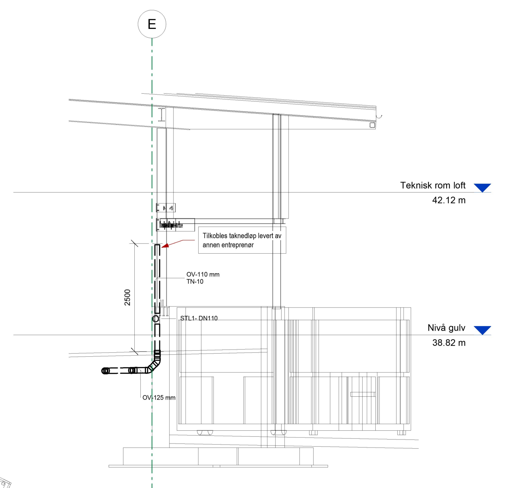
2 Prinsipp taknedløp1 1 : 50
