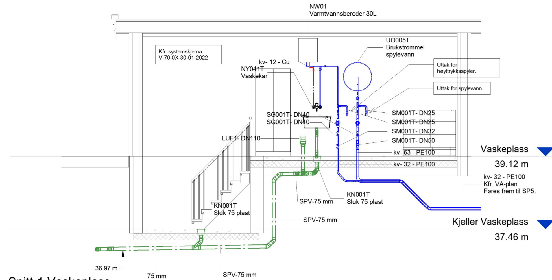
4 Snitt-1 Vaskeclass 1 : 50
