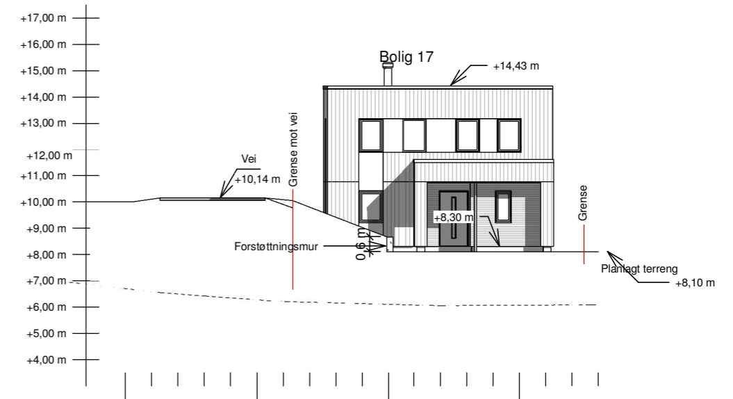
Terrengprofil 17-N 1 : 200
