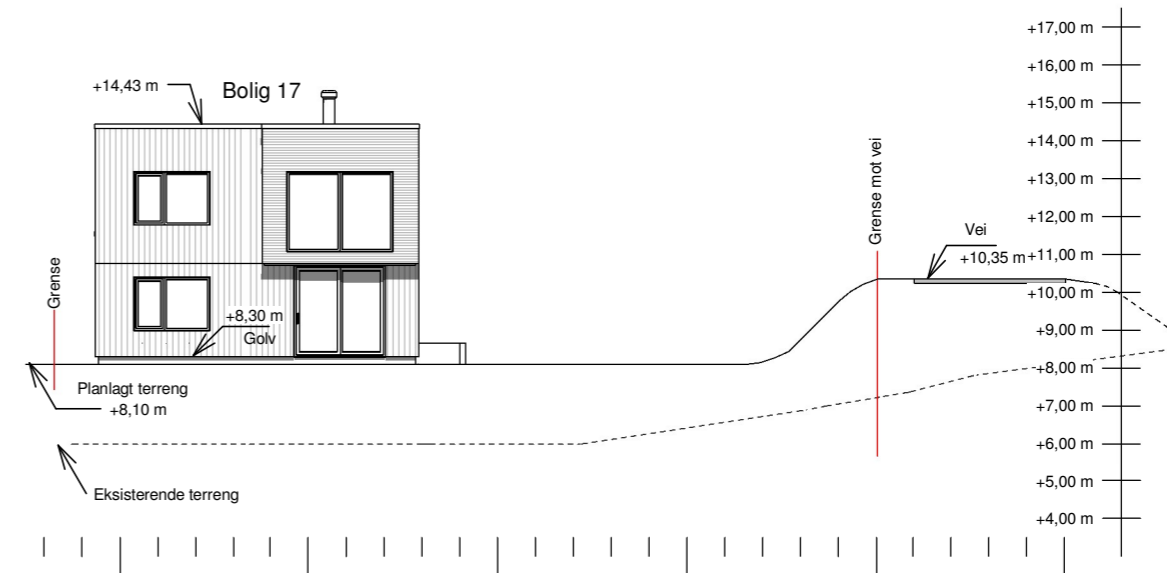
Terrengprofil 17-S 1 : 200
