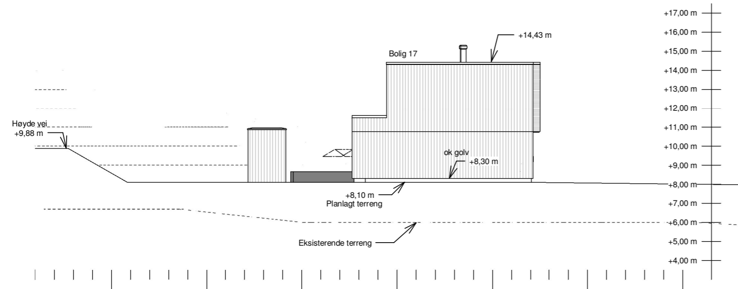
Terrengprofil 17-V 1 : 200
