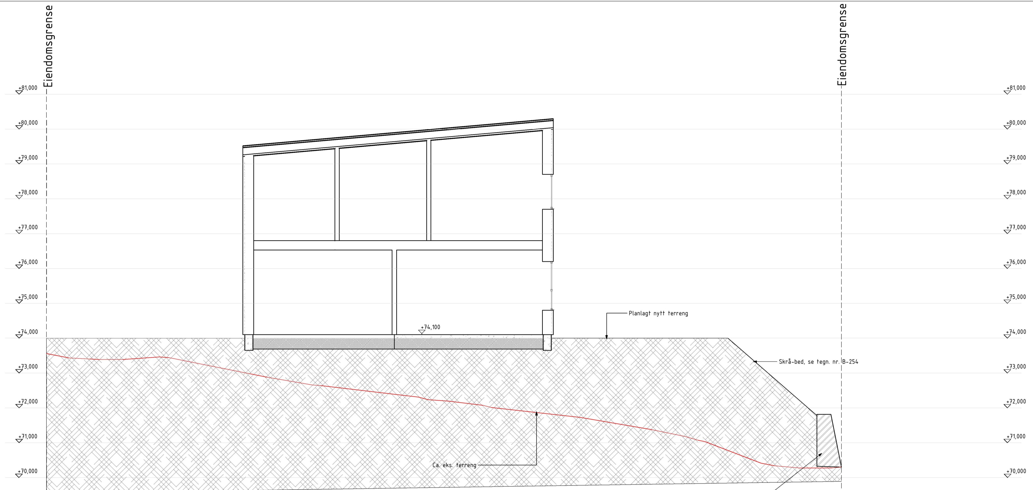
Terrenqsnitt 1 1 : 50
