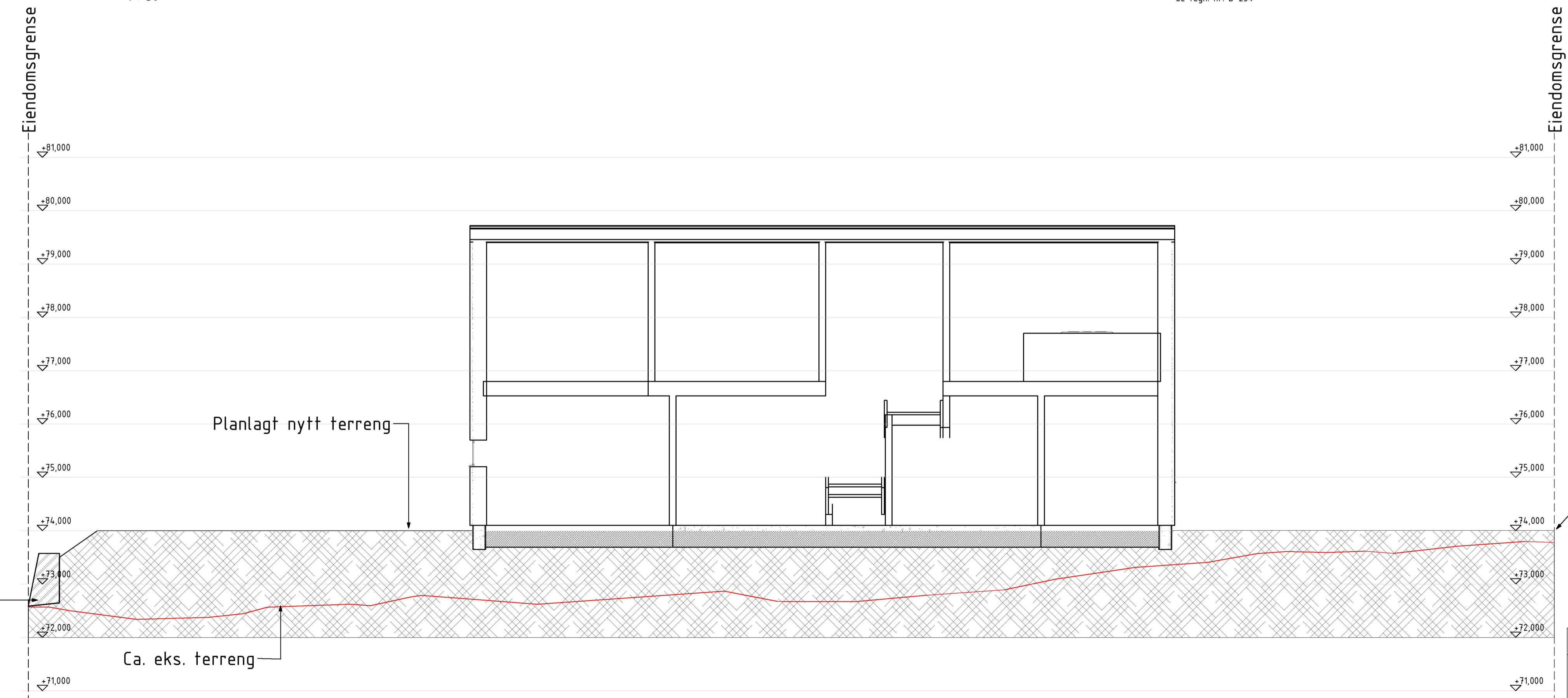
Terrenqsnitt 2 1 : 50
