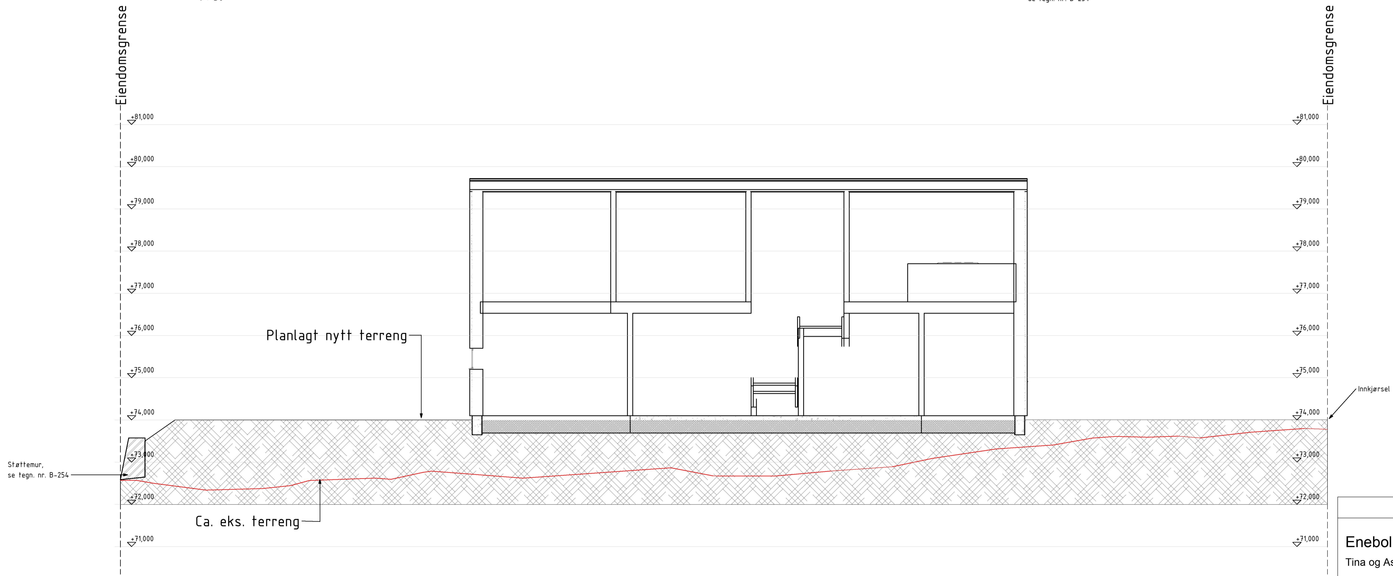
Terrenqsnitt 2 1 : 50
