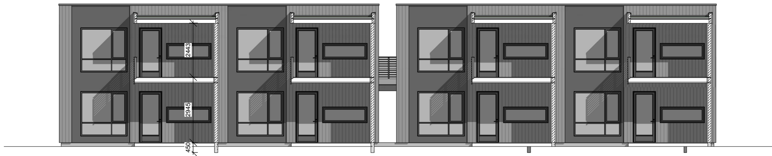
Snitt E 1 : 100
