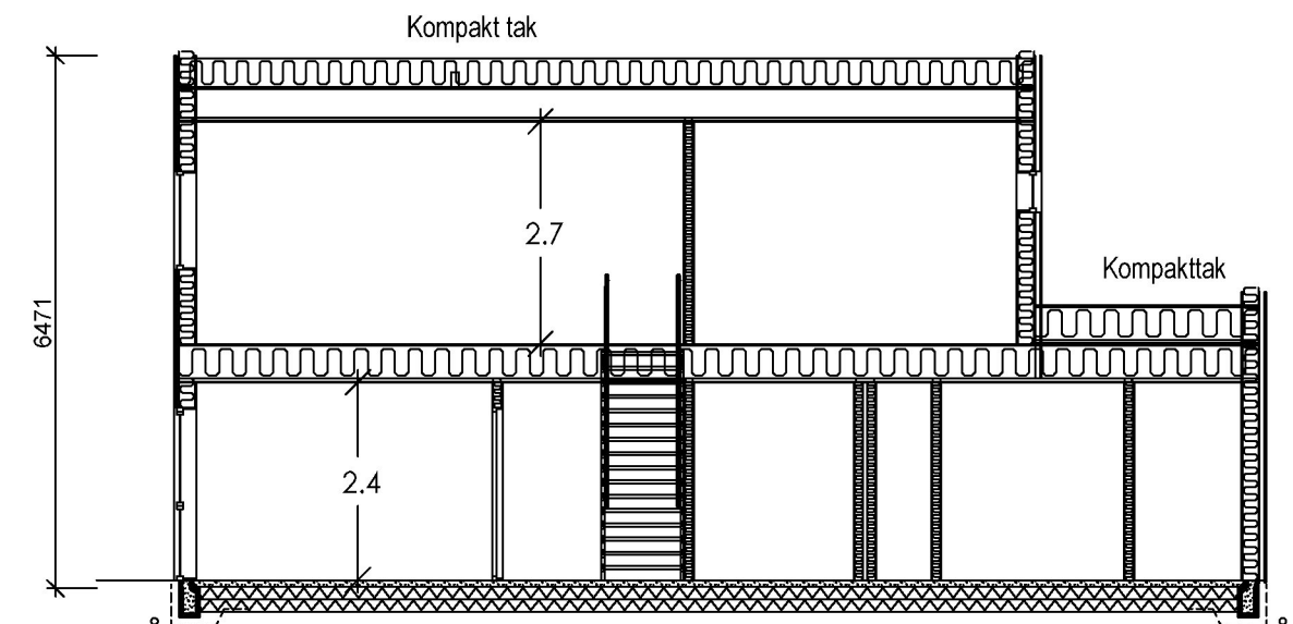
Snitt A:A
