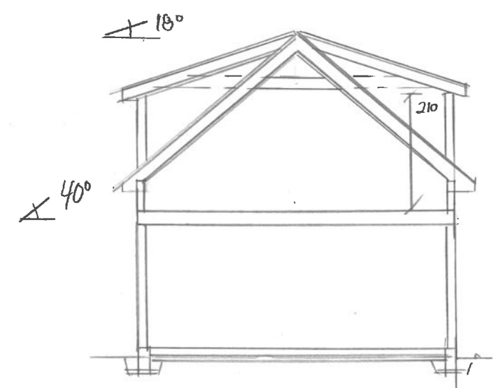
SNITT
