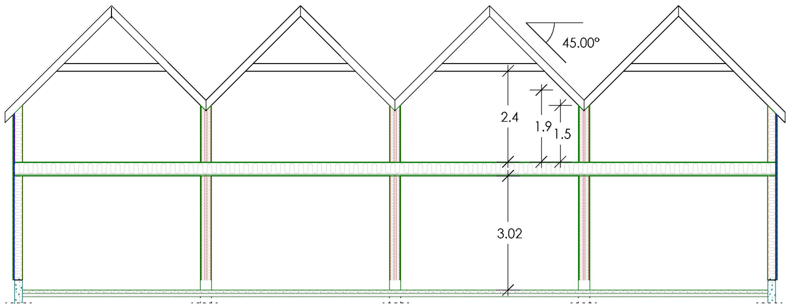
Snitt A-A
