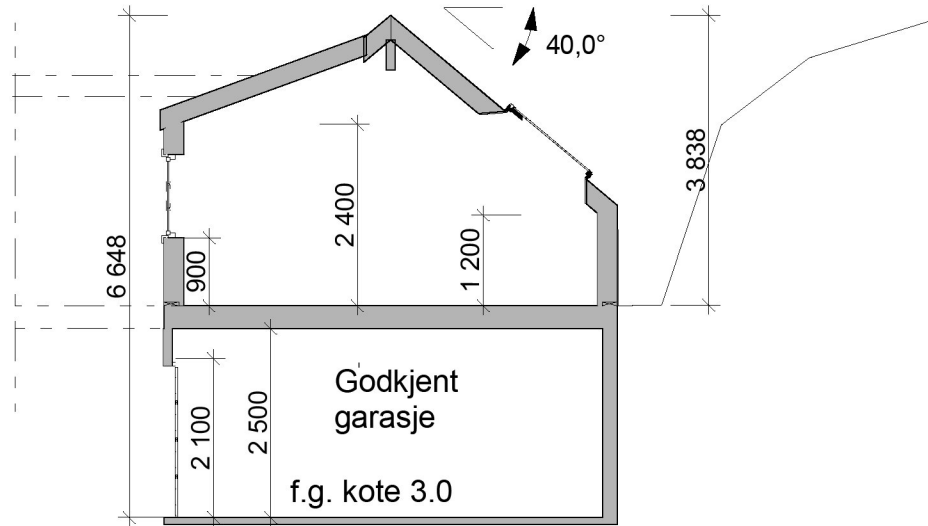
Snitt A
