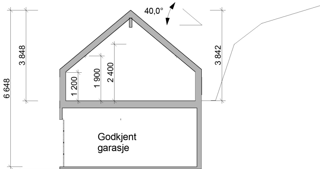
Snitt B
