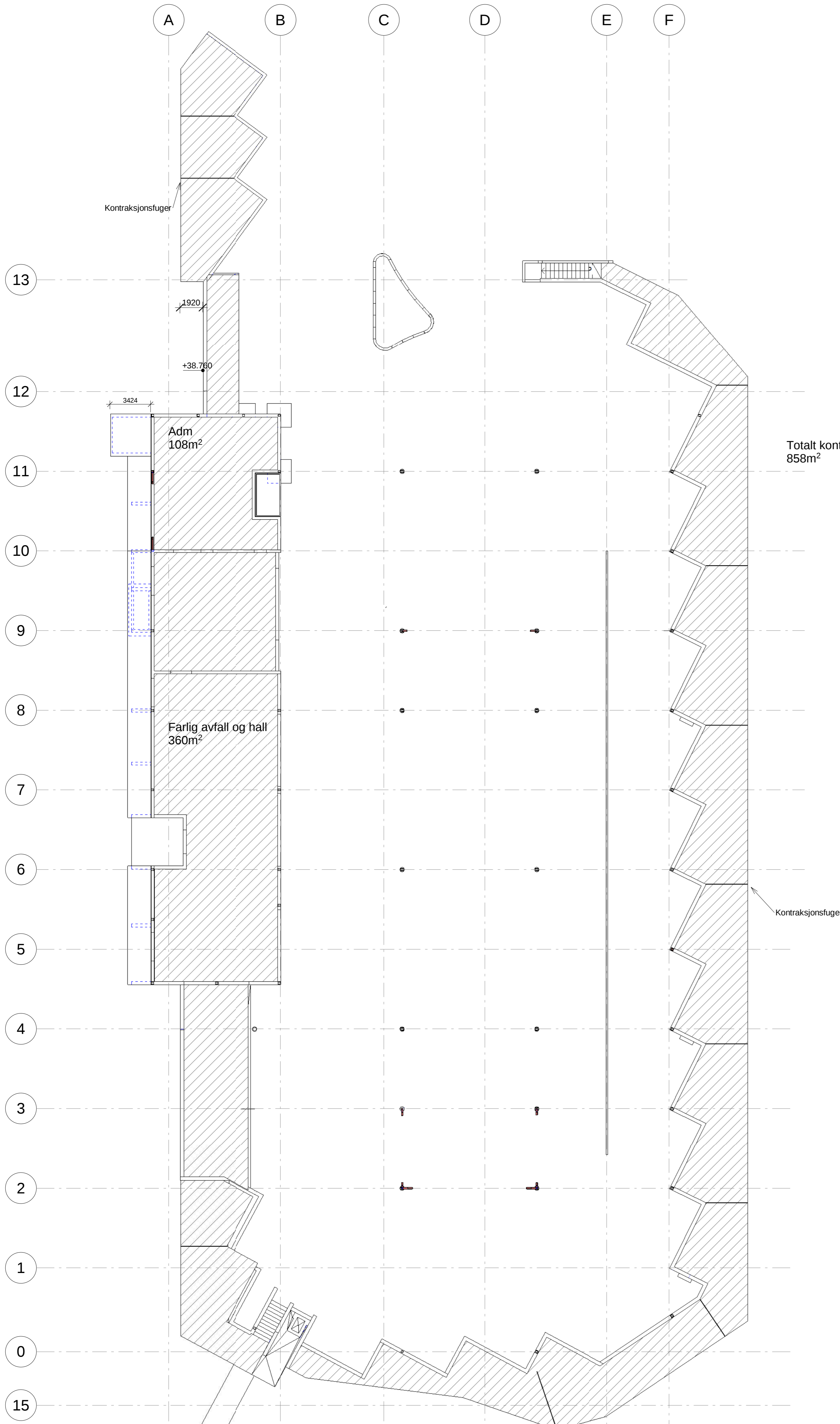
Arealer Betongdekker 1 : 200
