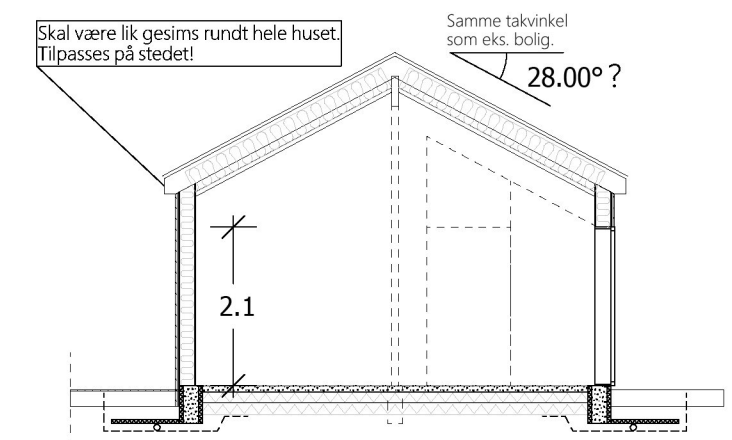
Snitt B-B
