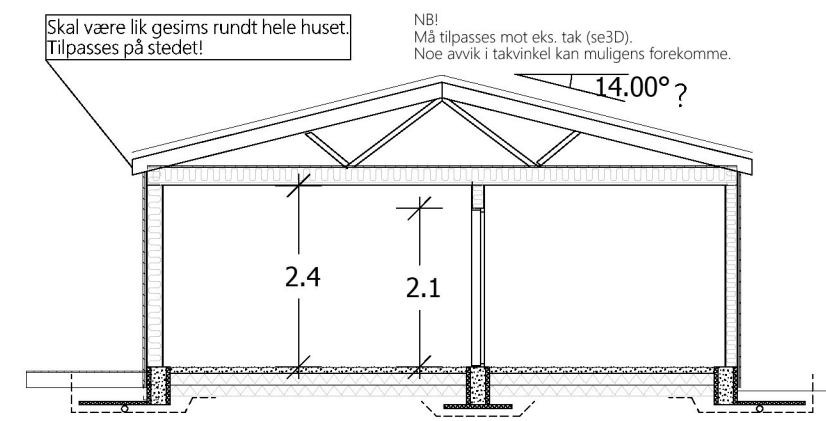
Snitt A-A
