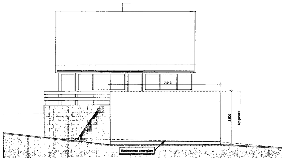
1:100 Fasade Sør
