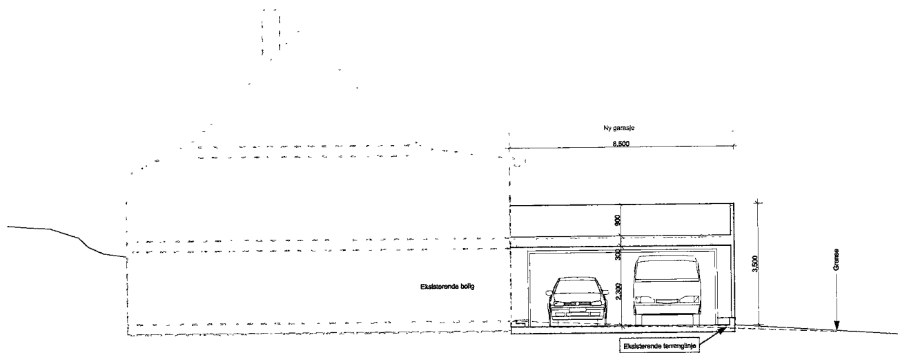
1:100 Fasade Vest
