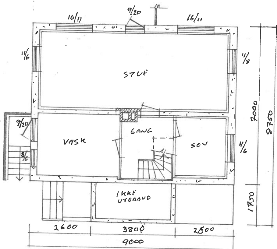
PLAN UNDERETASJE
