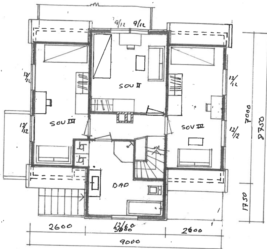
PLAN II-ETASJE
