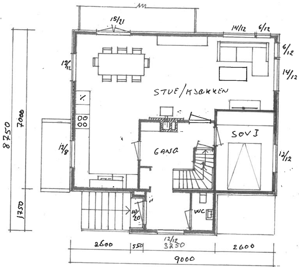
PLAN I-ETASJE
