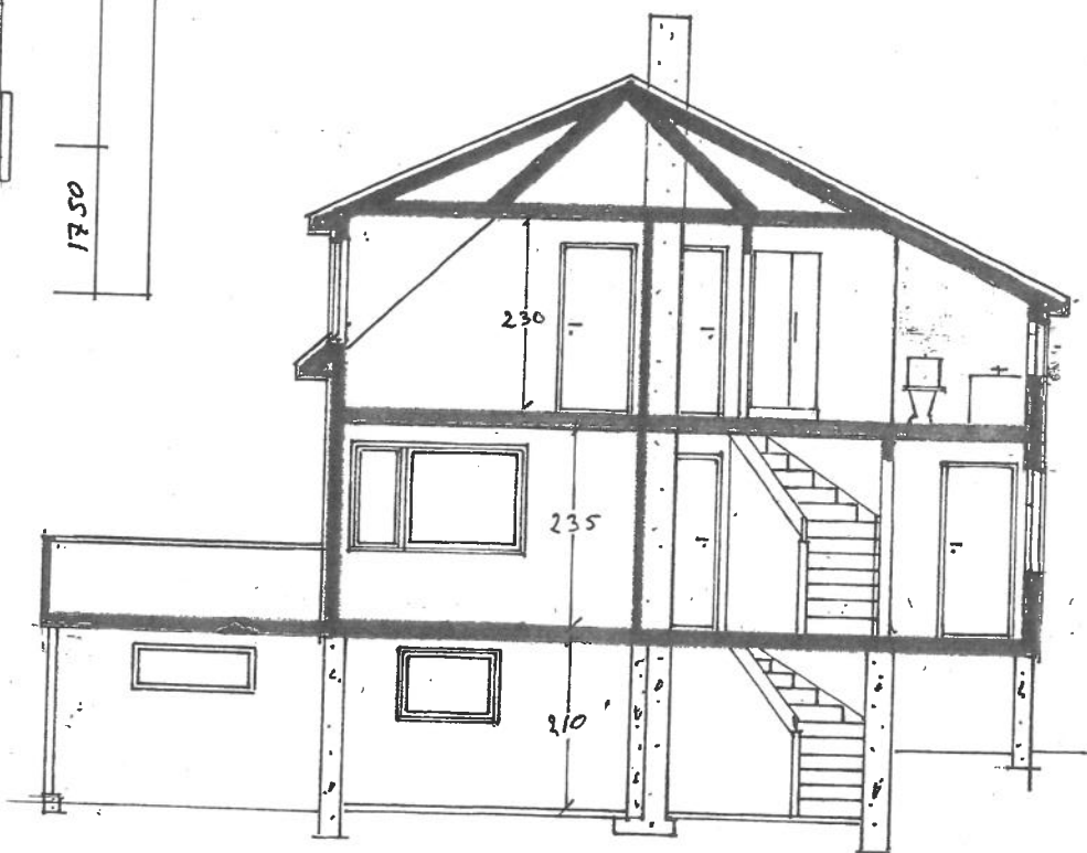
SNITT
