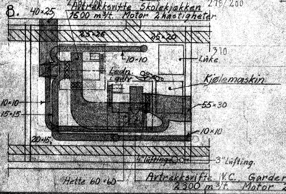
PLAN AV VIFTEROM PÅ LOFT OVER ROM NR. 308 OG 309
