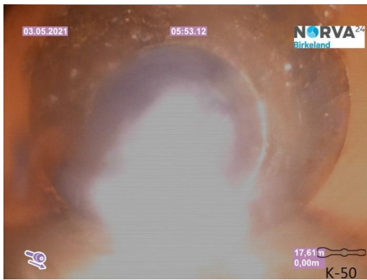
Spillvann_Stakeluke garasje_Påkobling_20210503_140725.jpg
