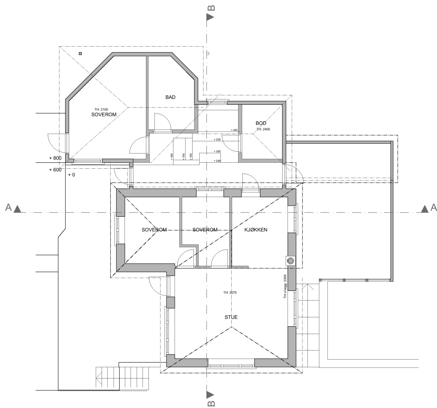
EKSISTERENDE 1. ETASJE
