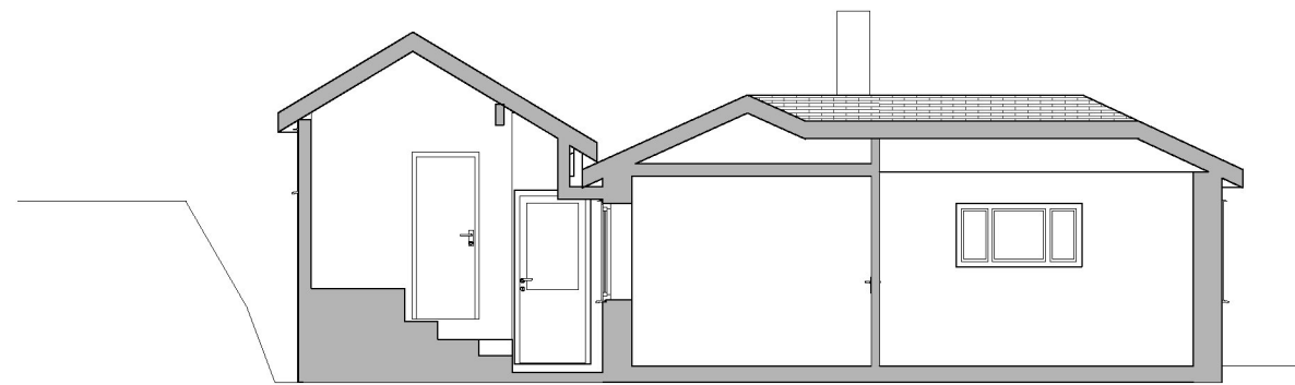
EKSISTERENDE SNITT B
