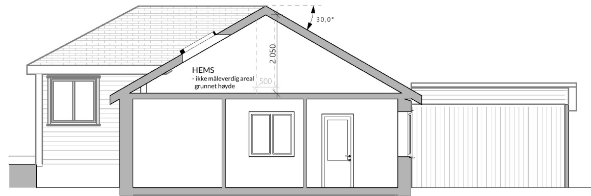
SNITT A
