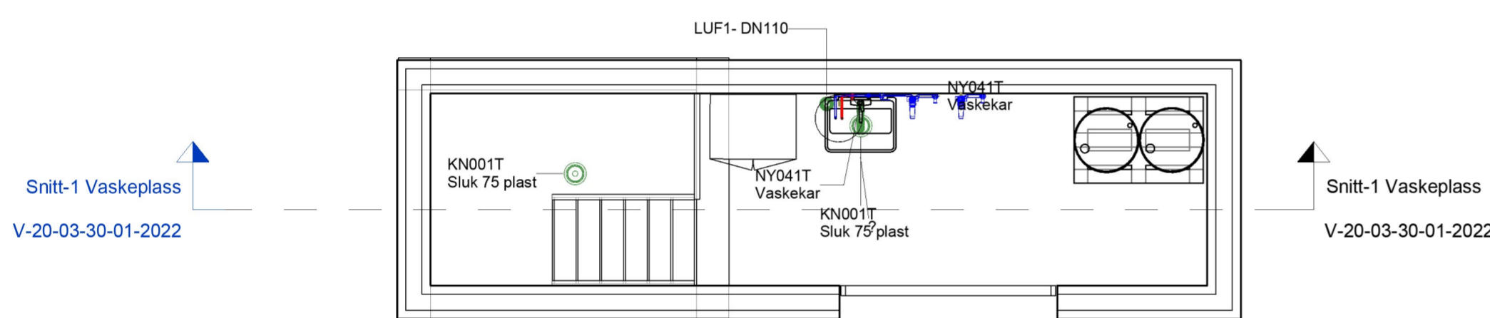
4 Snitt-1 Vaskeclass 1 : 50
