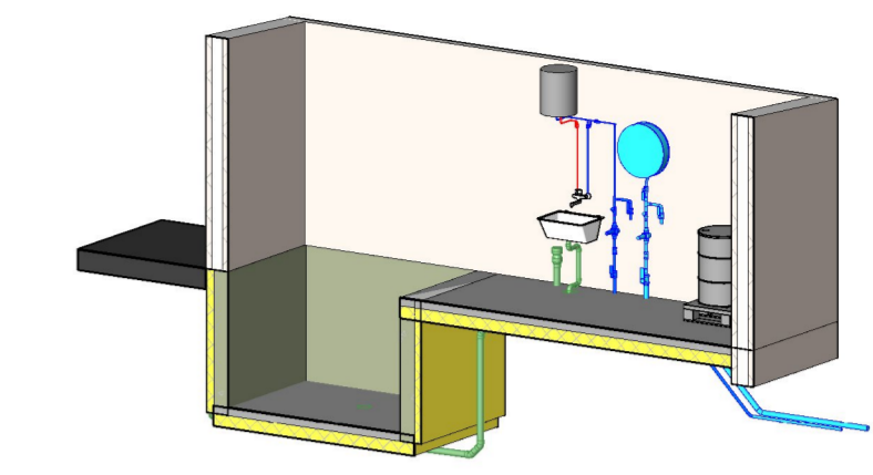
3 3D Vaskeclass
