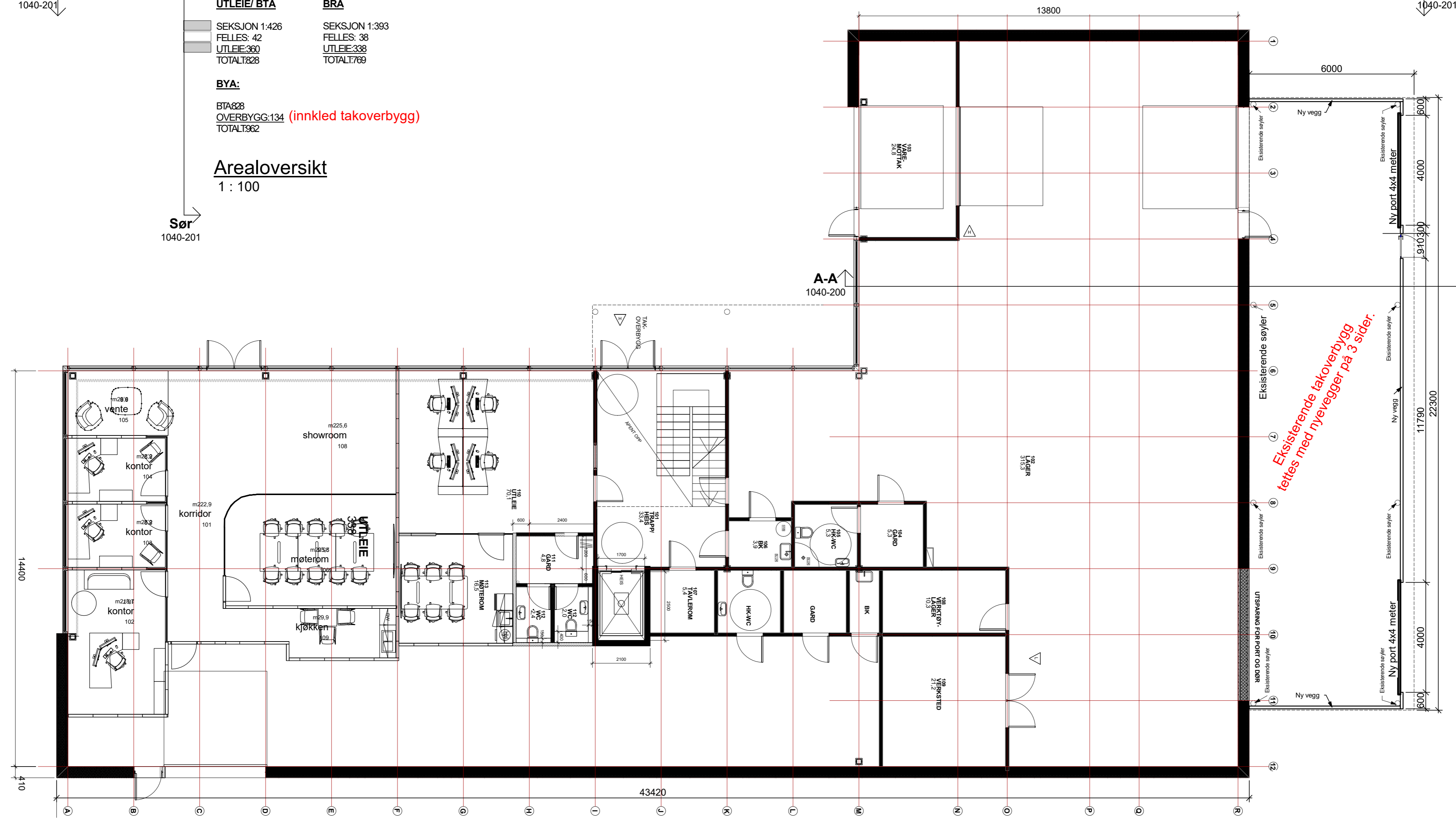
Plan 1. etg 1 : 100
