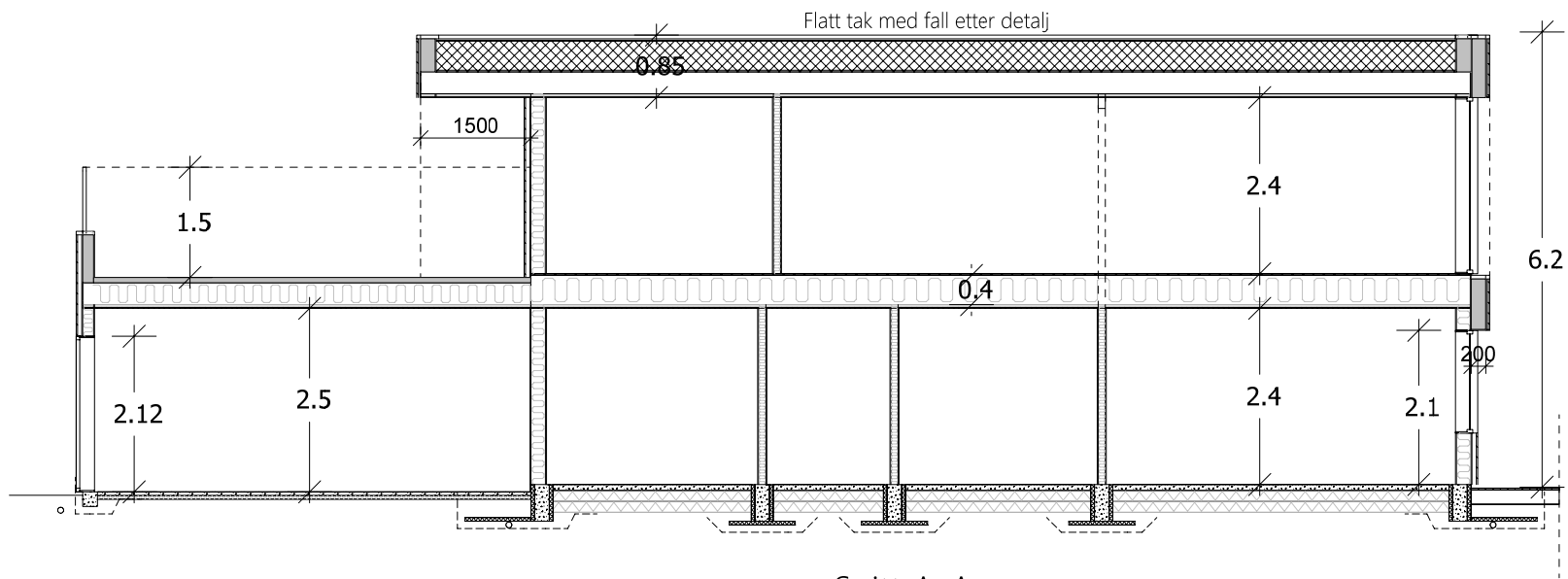
Snitt A-A
