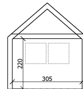
SNITT C-C
