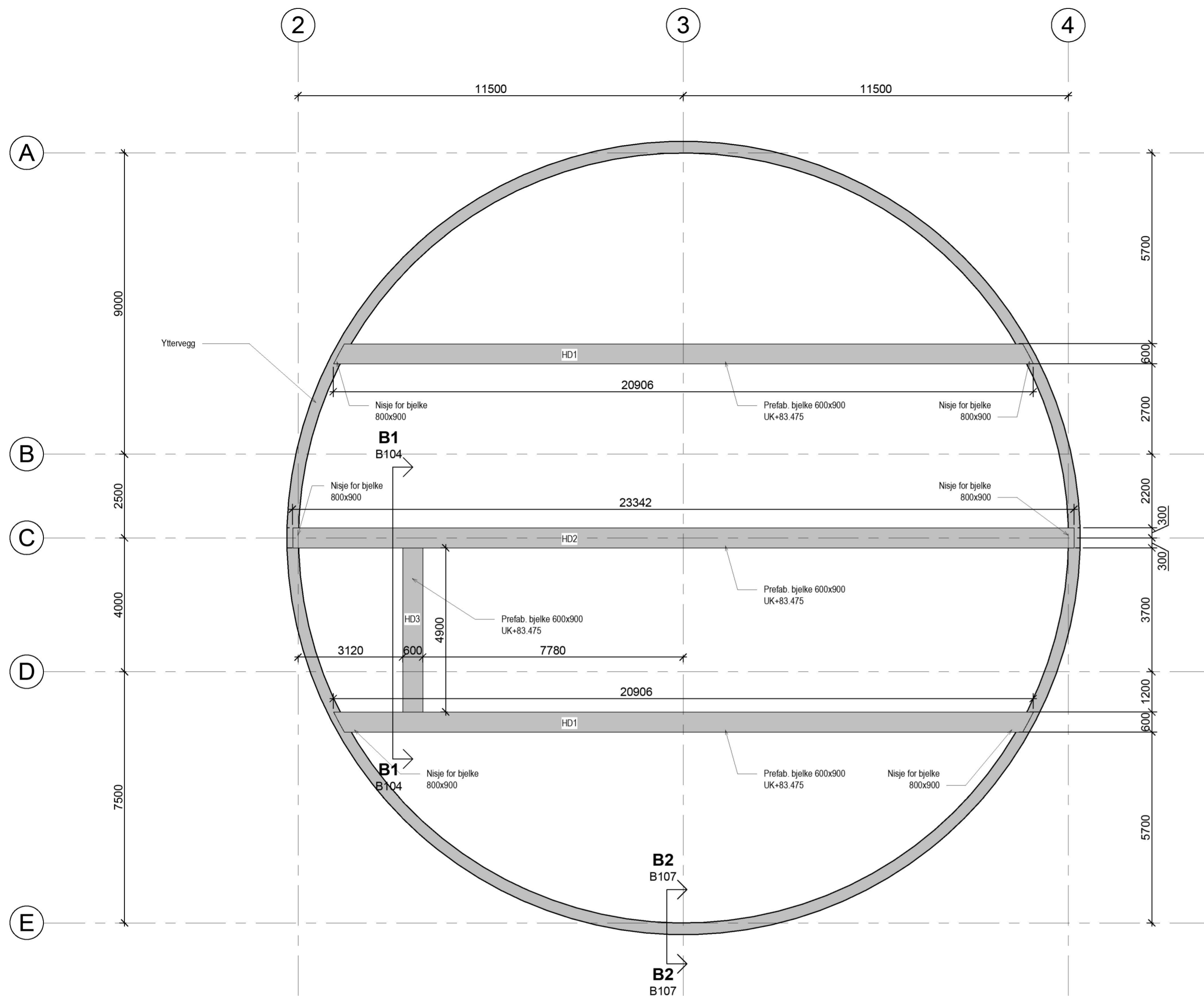
Takbjelkeplan 1 : 100
