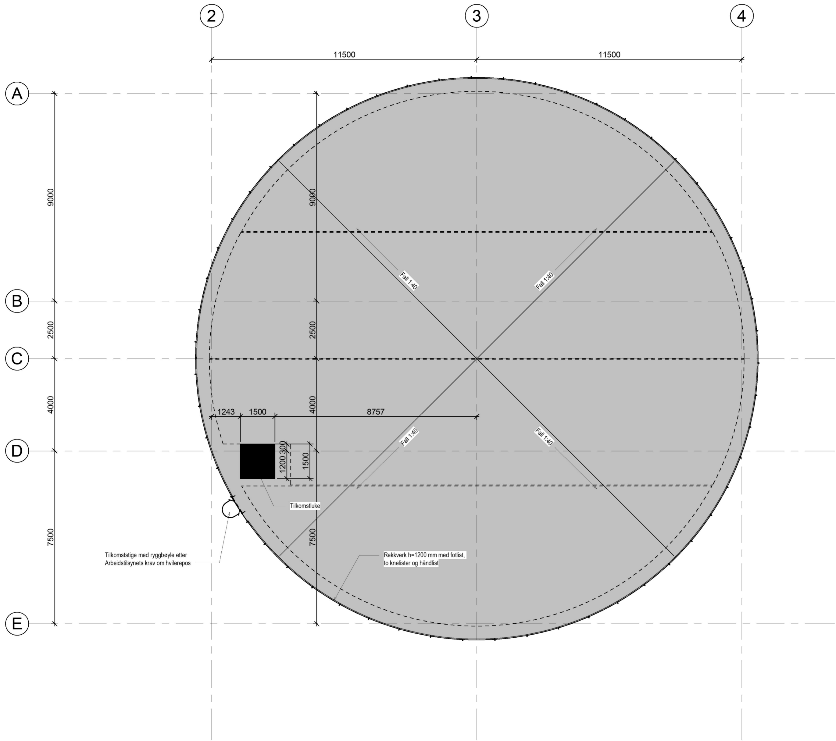
Plan 2 1 : 100
