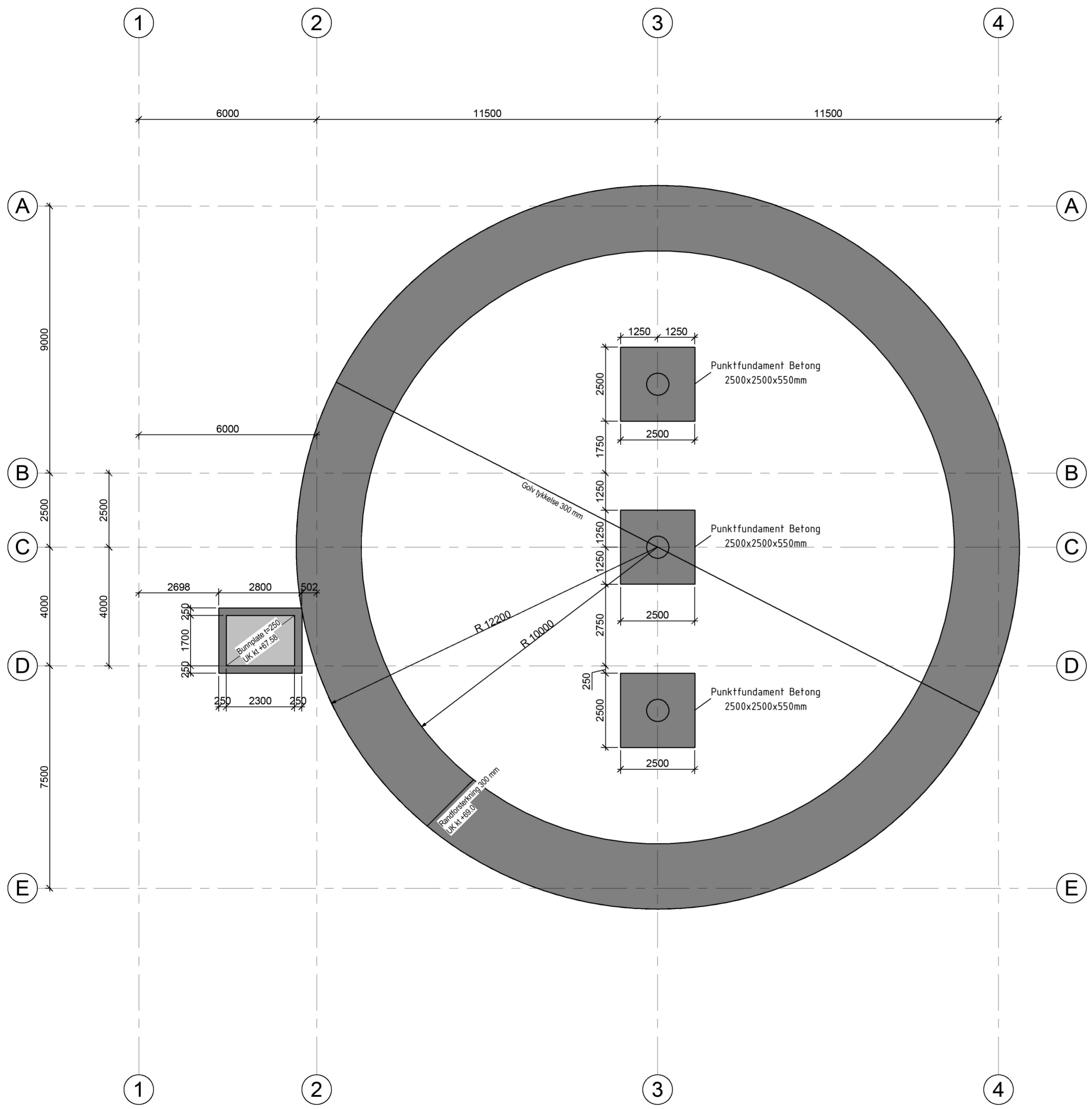
Fundamentplan 1 : 100
