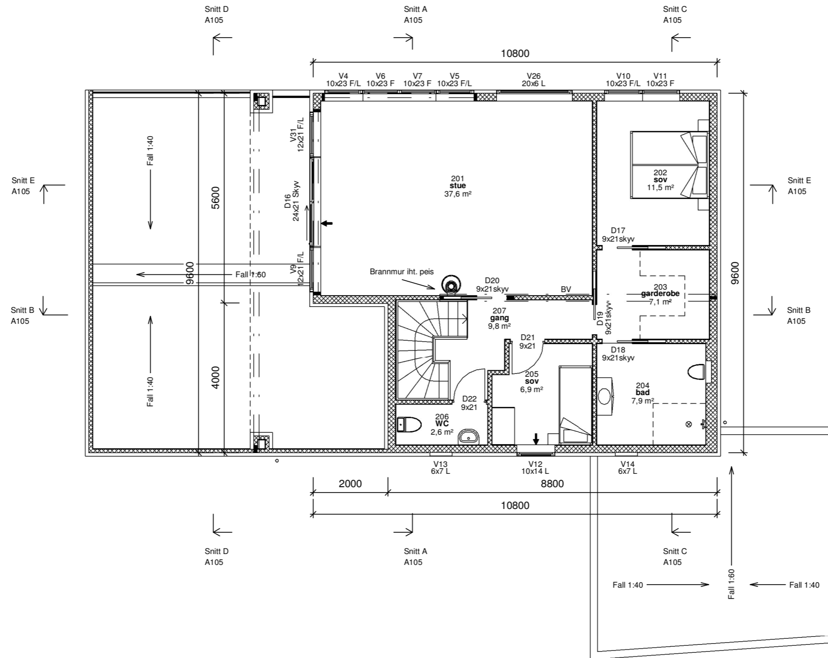
2.0 - 2.etasje 1 : 100
