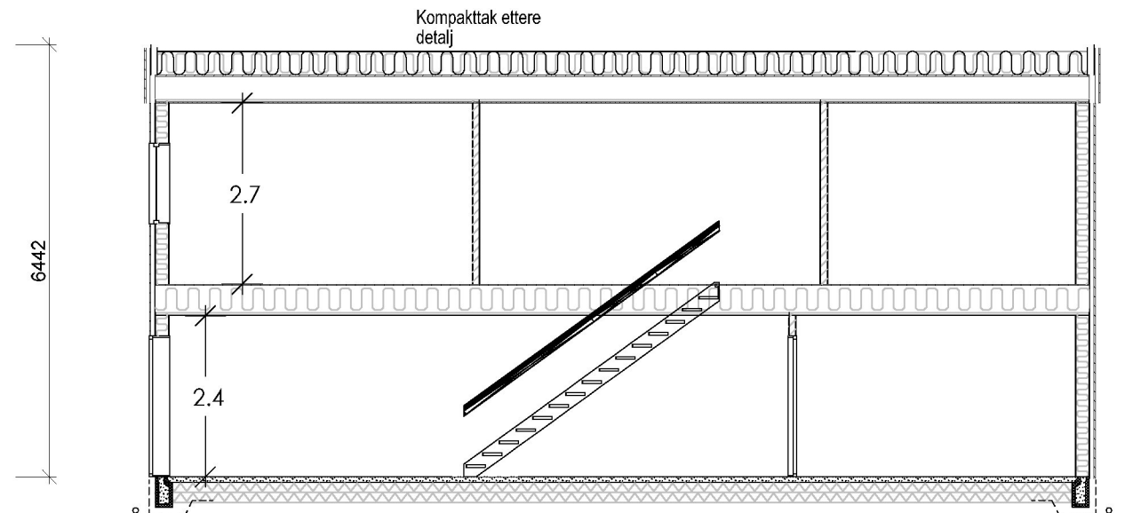
Snitt A:A
