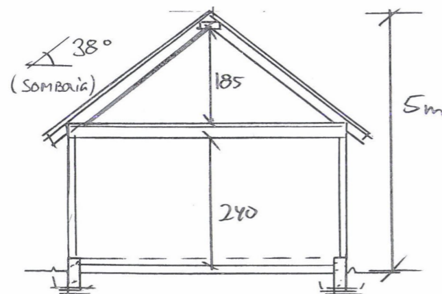
SNITT
