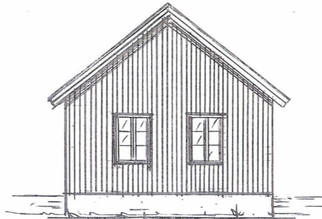
FASADE ØST
