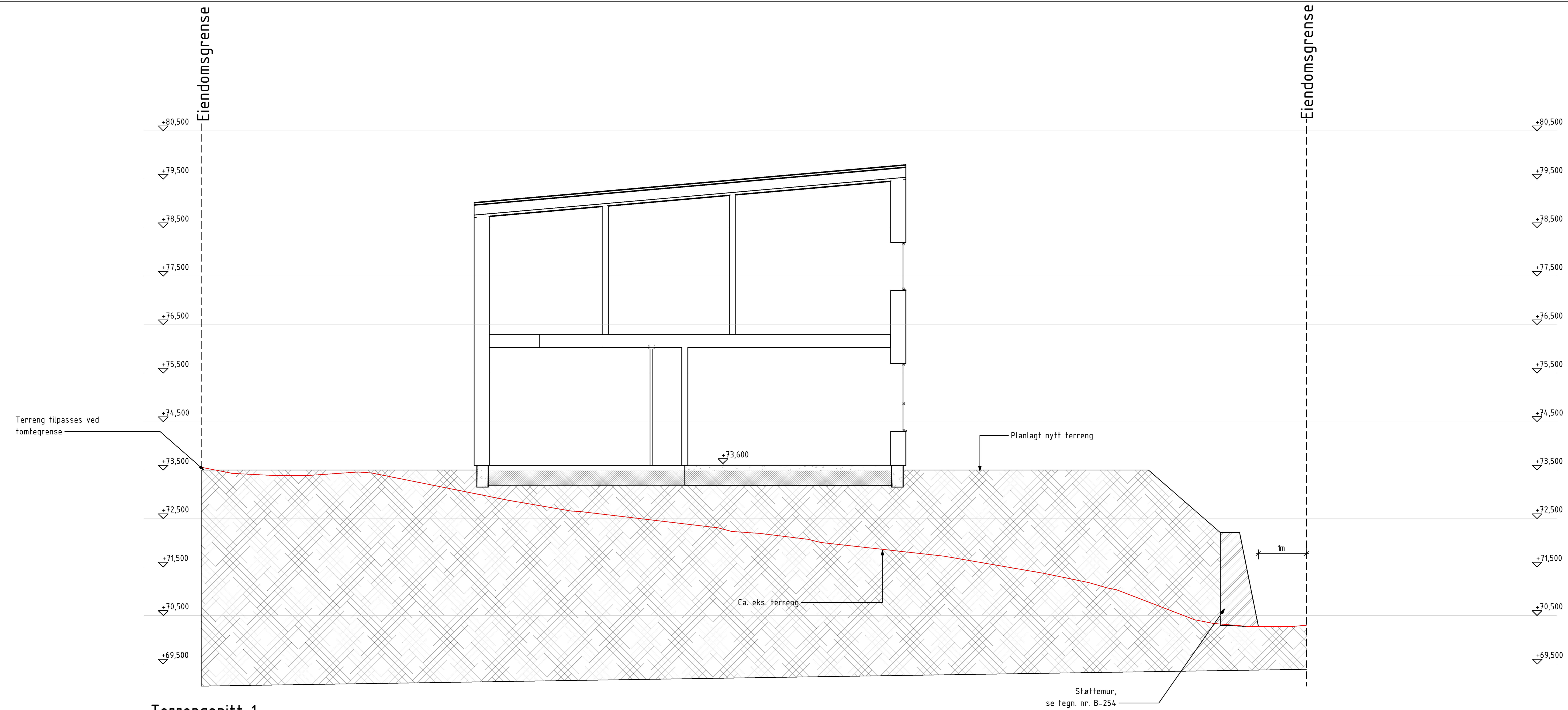
Terrenqsnitt 1 1 : 50
