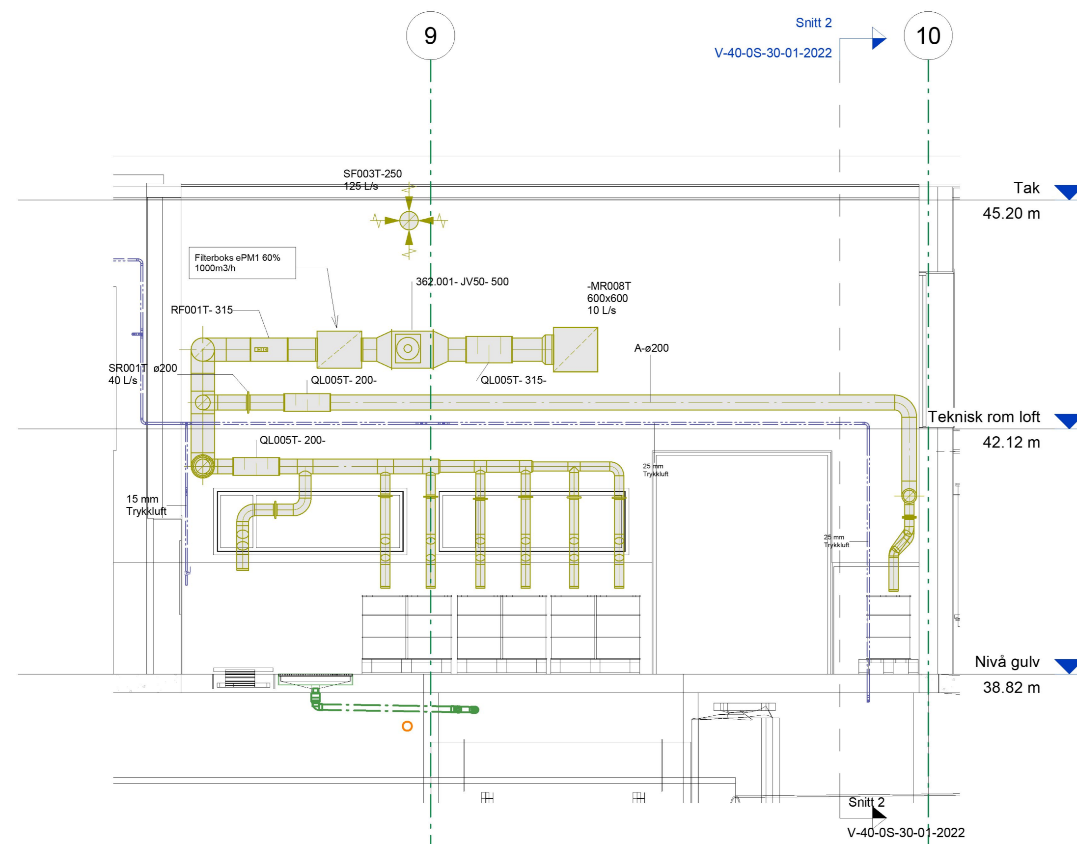
7 Snitt 3 1 : 50
