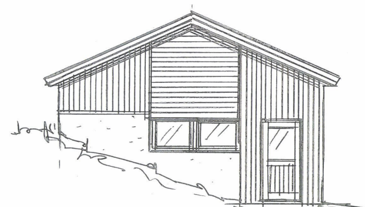
FASADE SØR
