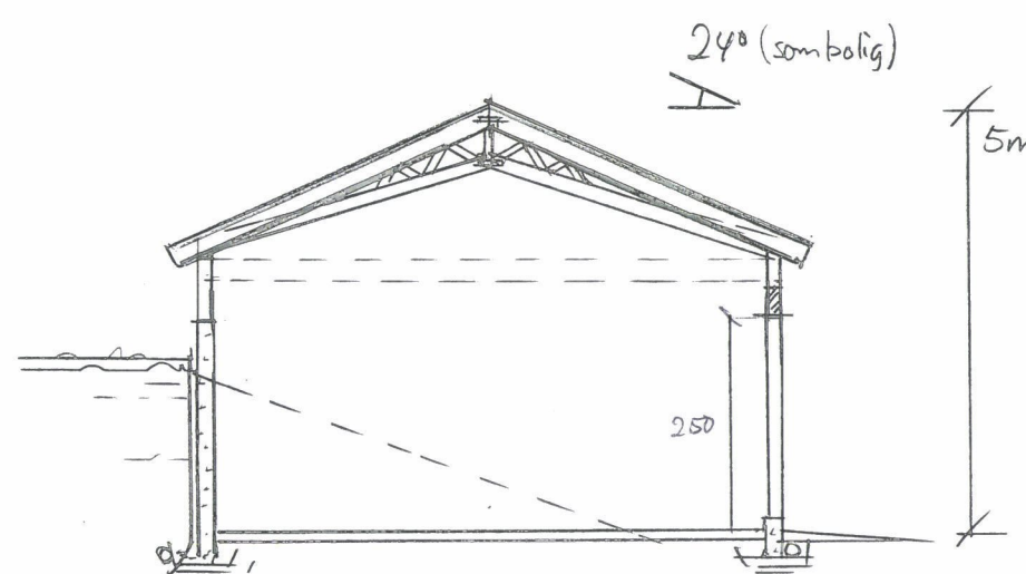
SNITT
