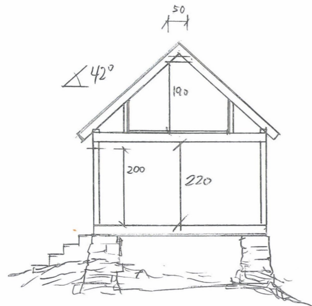
SNITT
